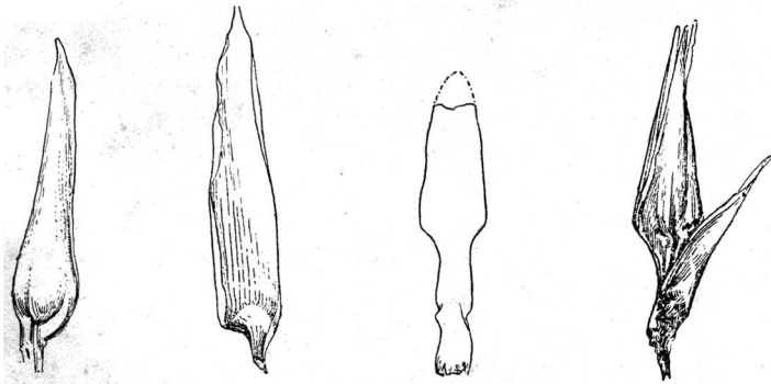
Puya Smithii Castellanos n. sp. Planta in natura (fide Schreiter). Sepalum facies exterior, interior, -\frac{2}{1} . Patalum \pm \frac{1}{1} . Flos et bractea florifera +\frac{1}{1} . Herbarium tucumanum n° 6616.
